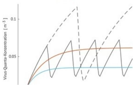
Theoretischer Verlauf der Viruskonzentration während einer Unterrichtszeit von 90 min für verschiedene Lüftungskonzepte (Grafik: Christian Schwarzbauer)
